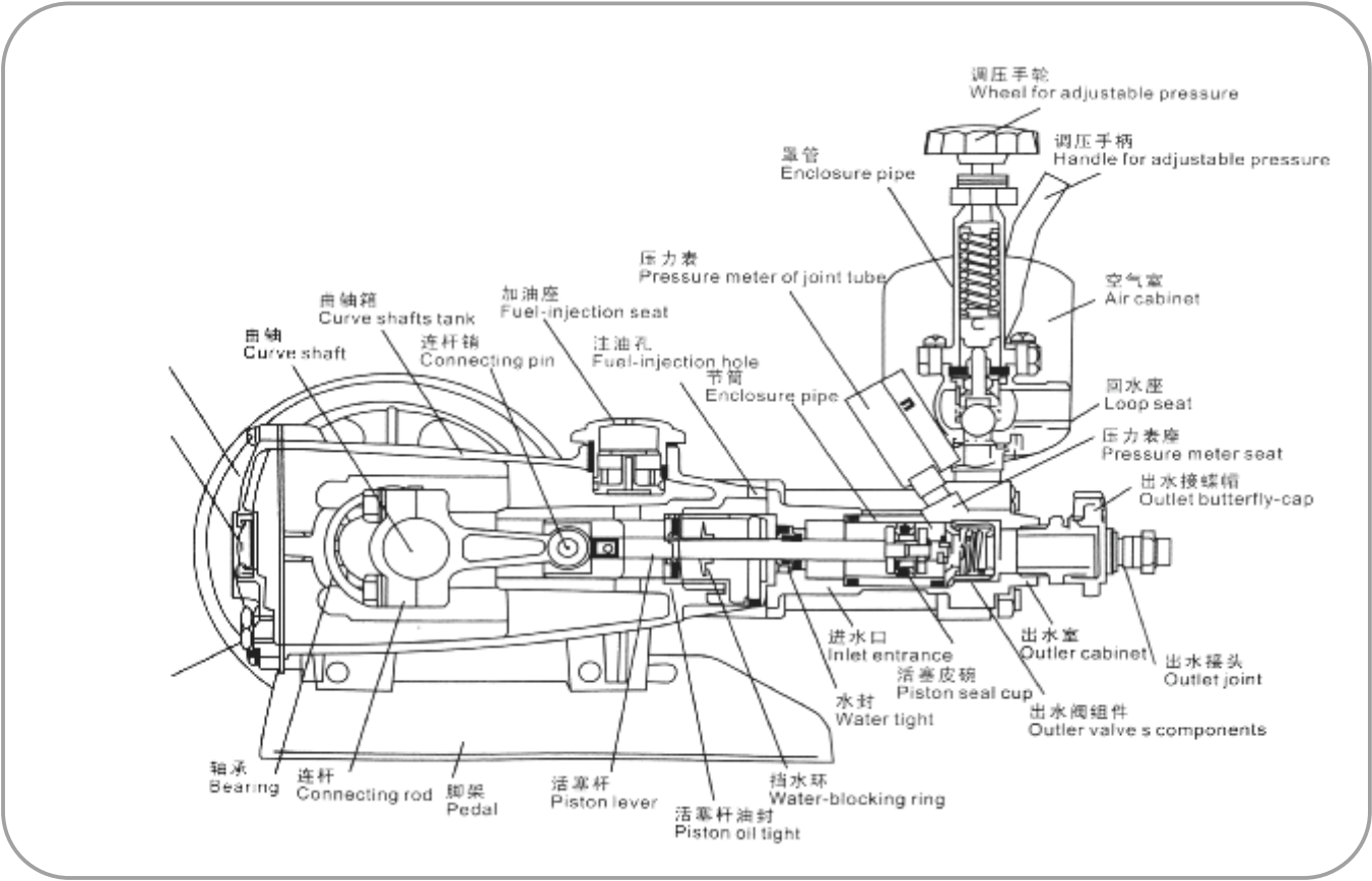
分解图 / Decomposition graph
